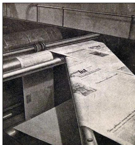
Role papíru v rotačce a skládající se stránky
