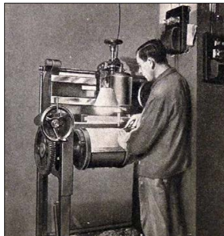
Frézovací stroj upravující nerovnost půlválce
