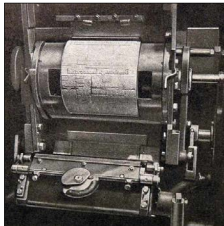
Detail odlitku půlválce pro tisk na rotačce
